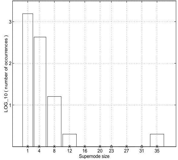
(d) Matrix 15: 7320 rows, 893 supernodes
