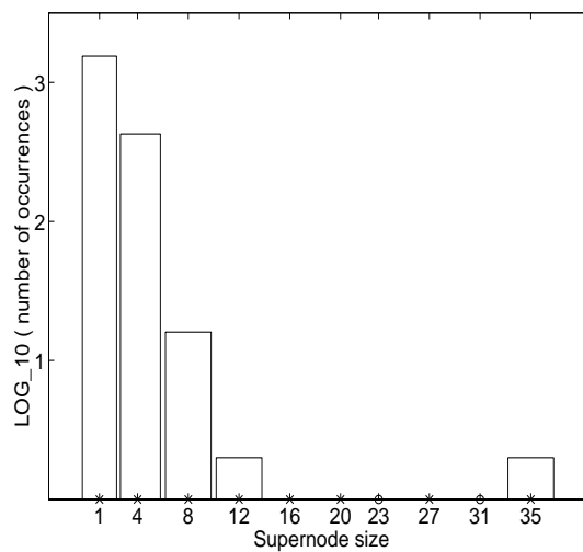
(d) Matrix 14: 7320 rows, 893 supernodes
